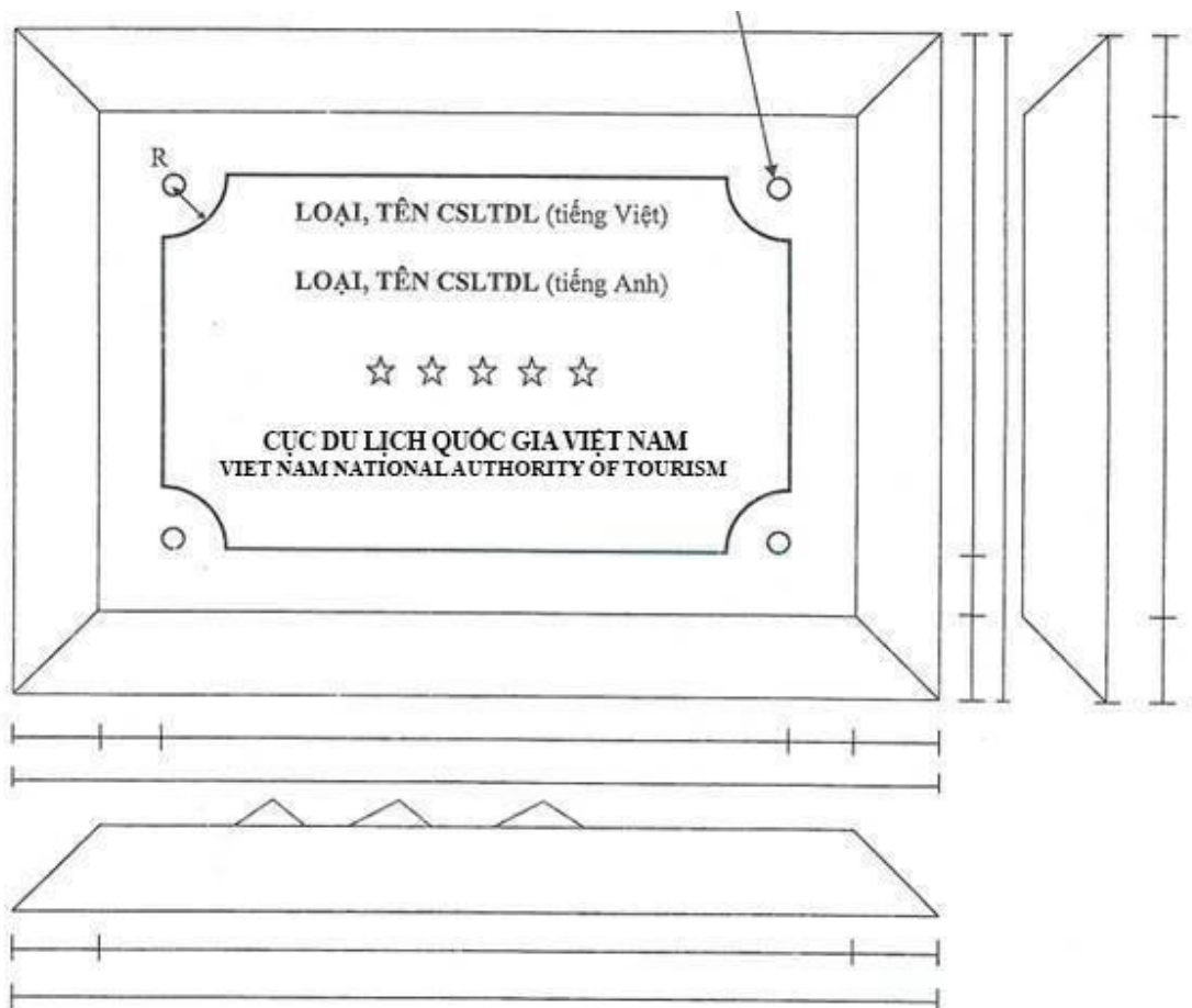
Hình 2: Mặt cắt ngang
