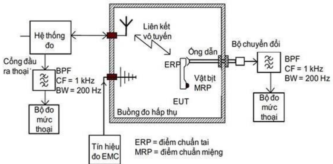
Hình 1 - Sơ đồ đo - Phương pháp giao thoa âm
